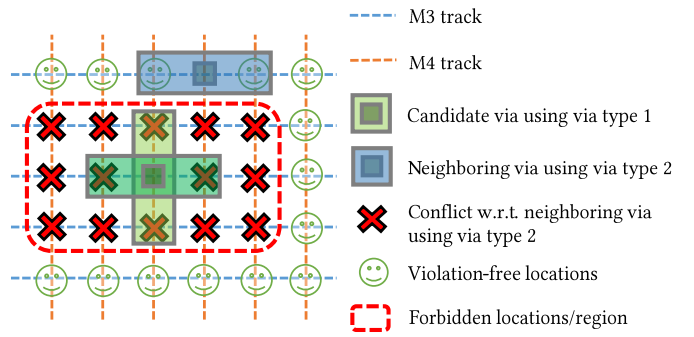
Fig. 7: Via-via LUT.
